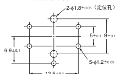
端子配置/内部连接图 （TOP VIEW）
