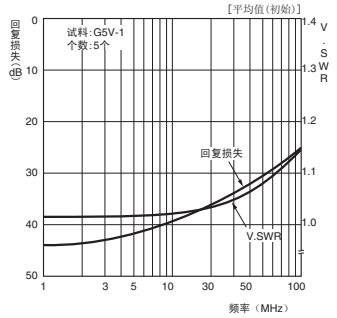
高频特性（回复损失、V.SWR）*1、*2
